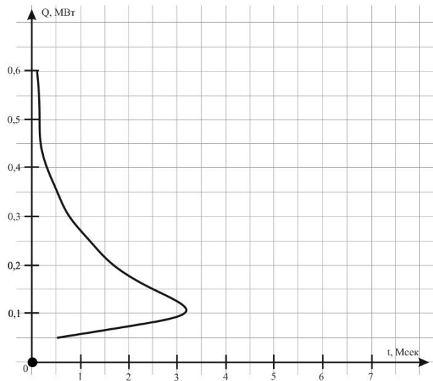
Рис. 2. График средних значений продолжительности отопительной нагрузки по 15 городам [4]
