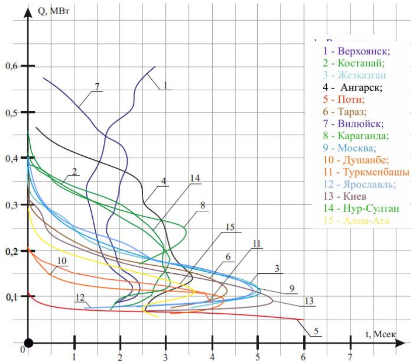
Рис. 1. Годовые графики продолжительности отопительной нагрузки 15 городов [3,4]
